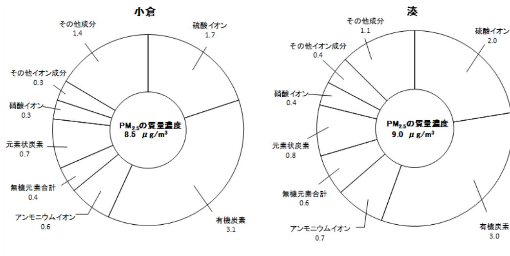
微小粒子状物質成分分析結果
