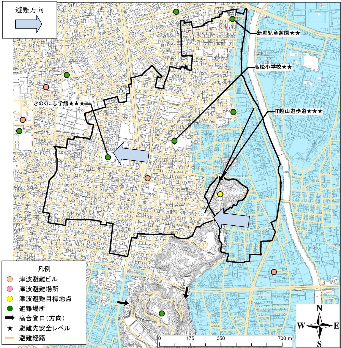
図 7 避難経路図
