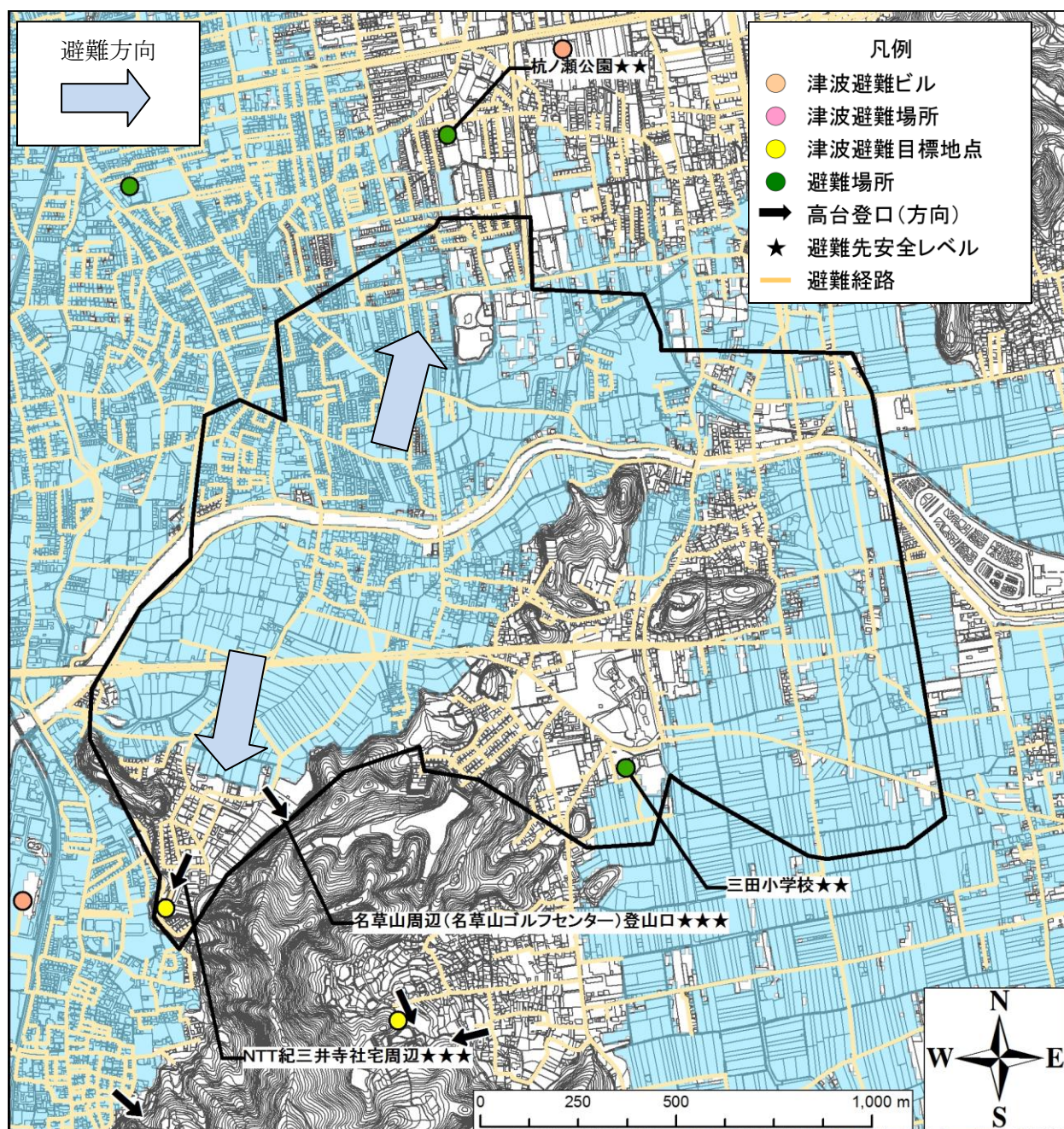
図 2-2 避難経路図
