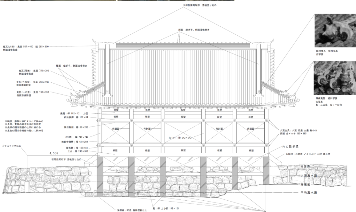
↓ 観海閣 東立面図
