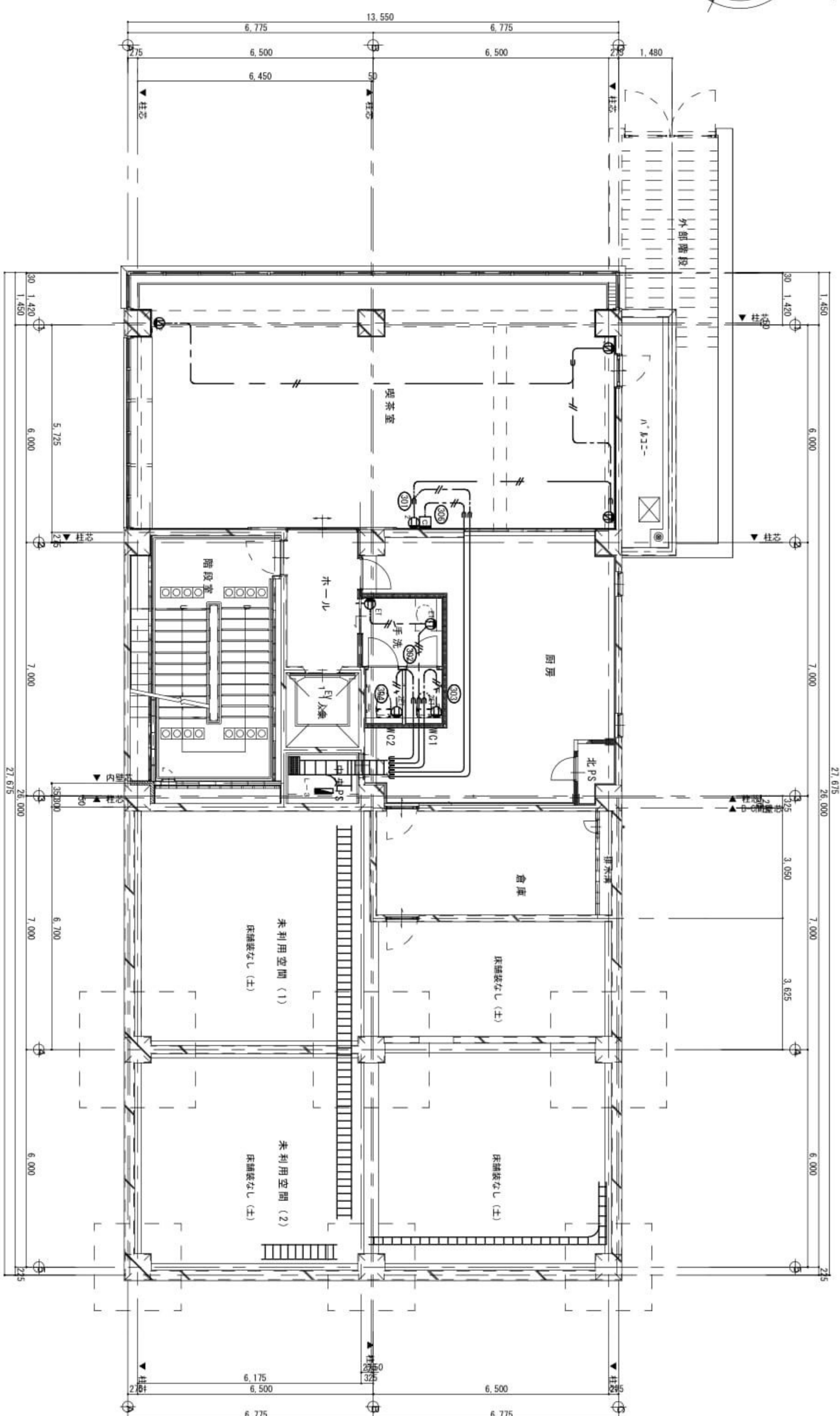
4階平面図 SCALE=1:100
