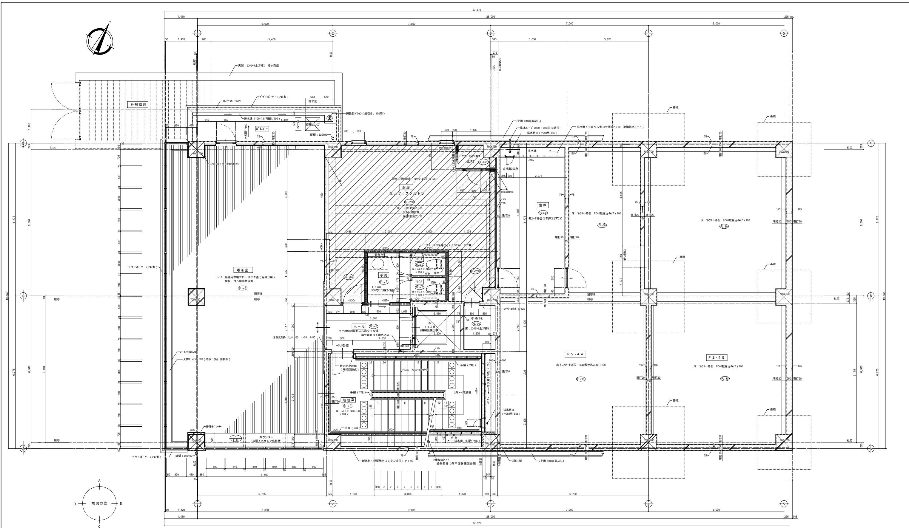
4階平面詳細図 SCALE = 1 : 50 厨房床部分：33'・250部分を示す
