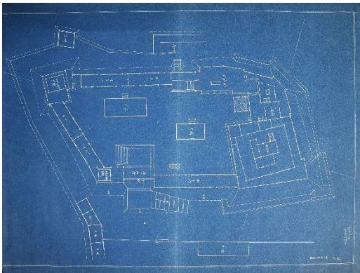
わかやまじょうてんしゆかくえ ずうつし 和歌山城天守閣絵図写【和歌山城整備企画課蔵】 嘉永二年（1849）西十一月朔日の銘が入った和歌山城天守閣図の写し。
