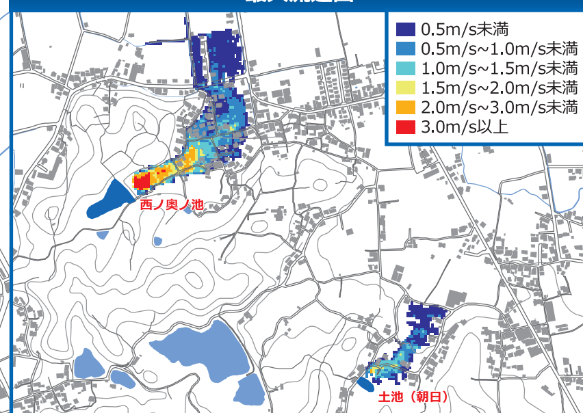
最大流速図
