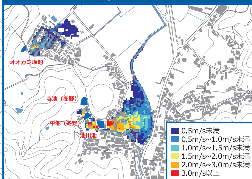
最大流速図
