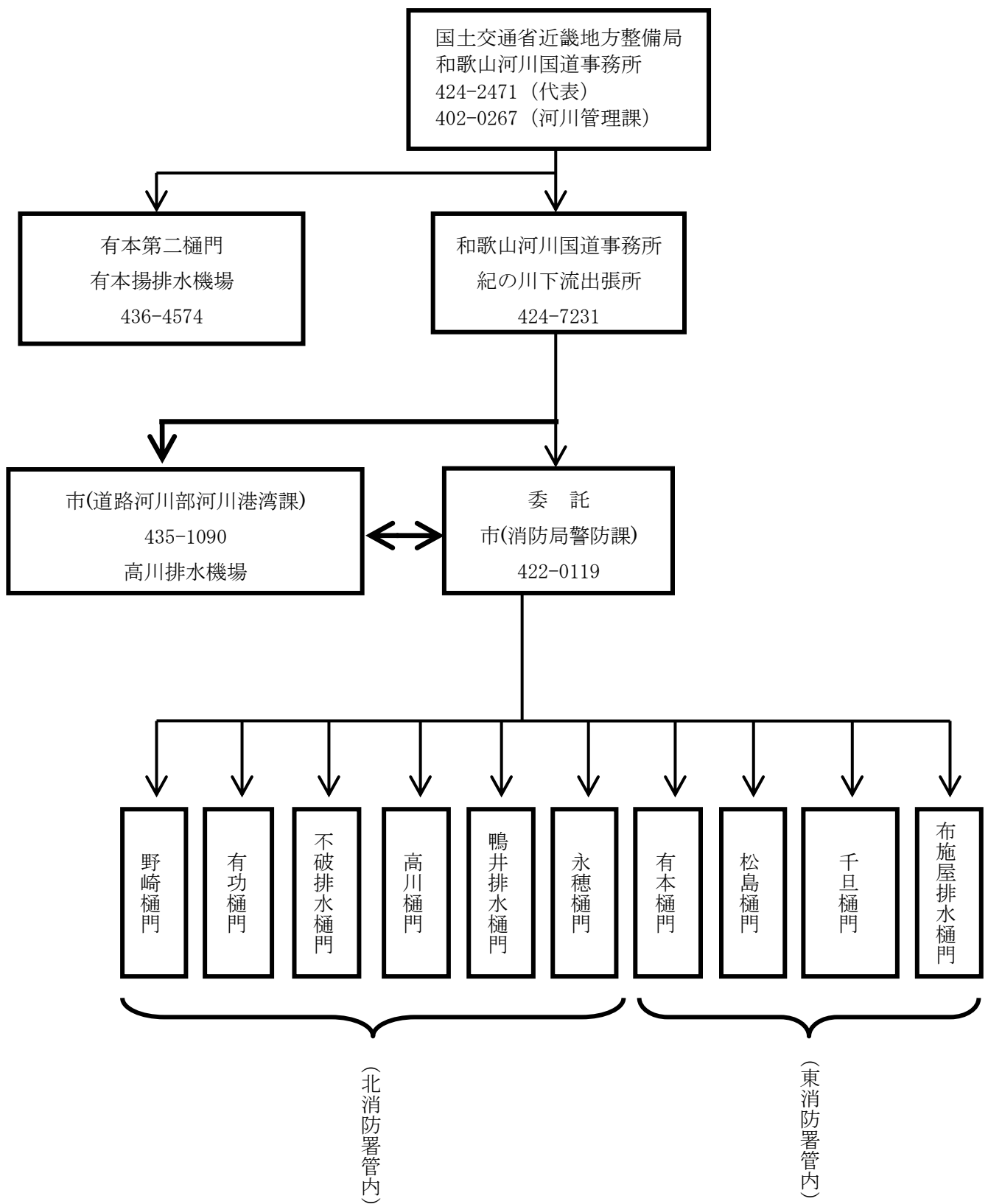
<紀の川水系樋門操作伝達系統図>
