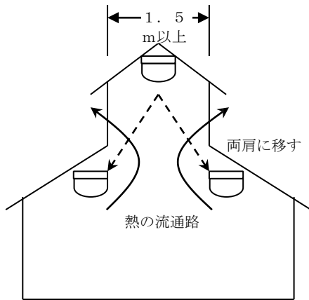
第24-43図 (断面図)
