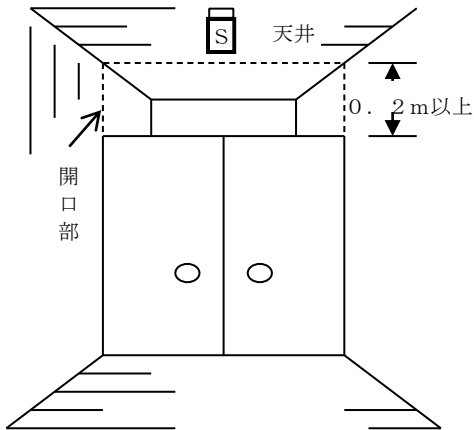
立面図
