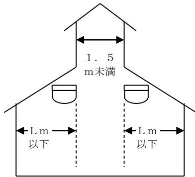
第24-42図 (断面図)
