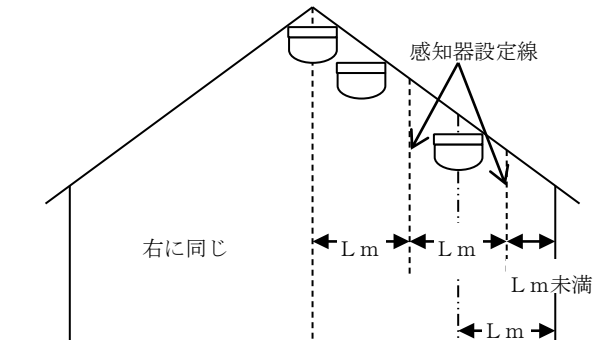
第24-38図 (断面図)
