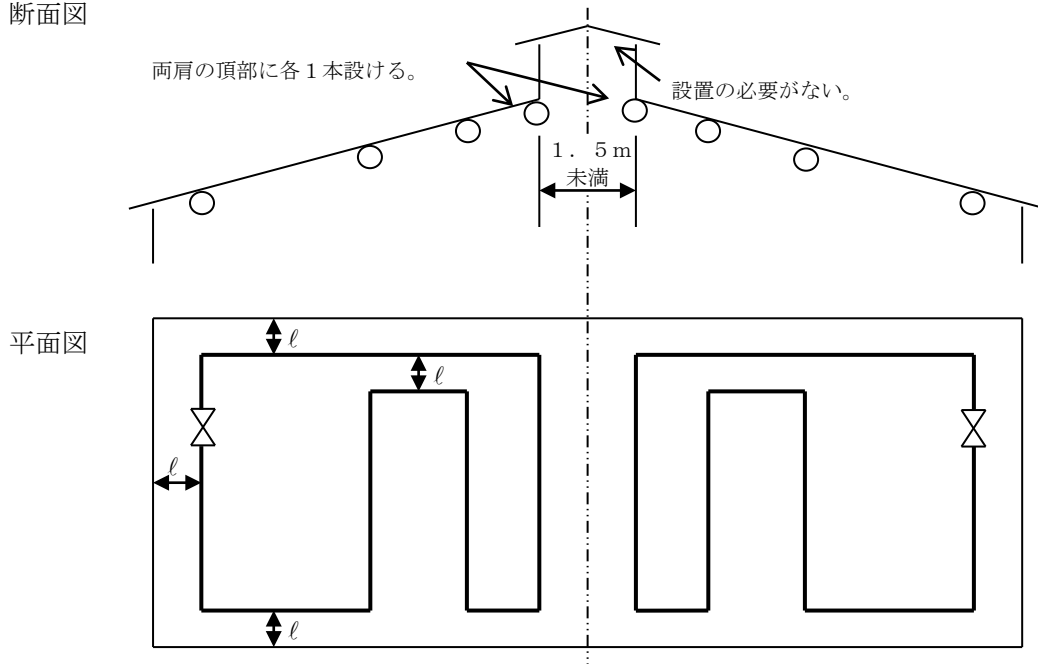
第24-88図 断面図
