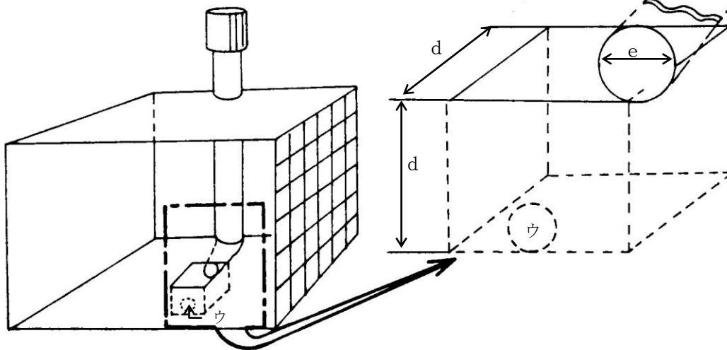
例図2 一ためますを整備室の中央に設ける場合の例一
