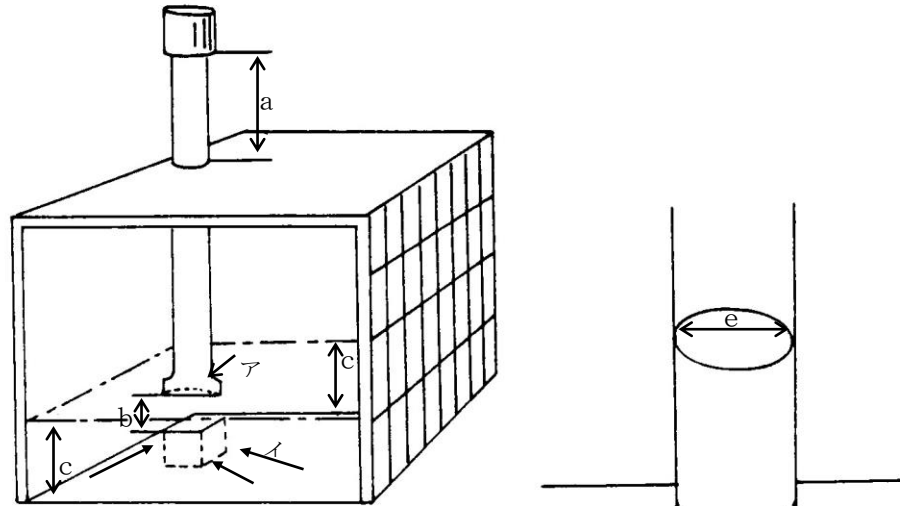
例図1 一ためますを整備室の隅に設ける場合の例一
