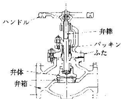
玉形弁の例
