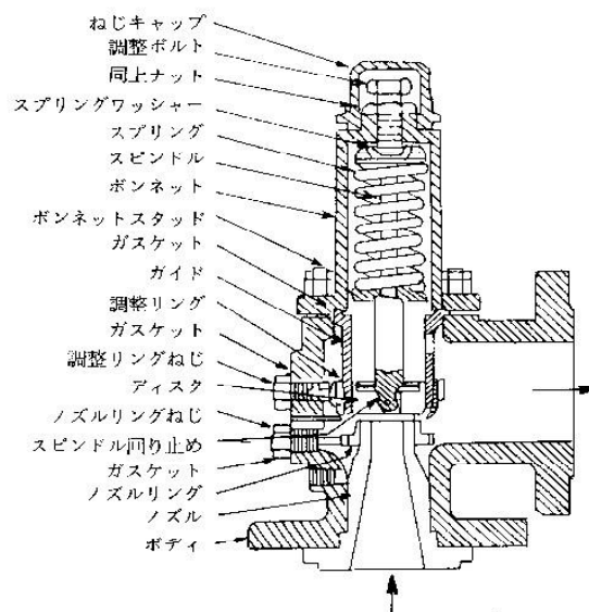
安全弁の構造例
