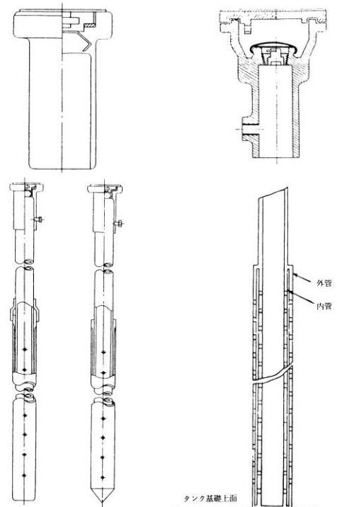
漏えい検査管の管体構造例
